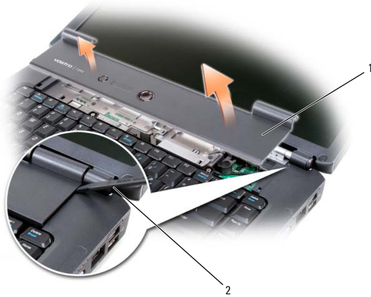
1 غطاء المفصل 2 المسمار
