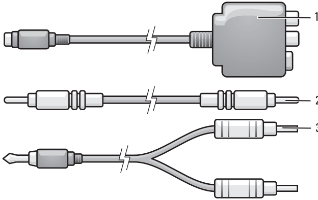
1 محول فيديو مركب 2 كبل الفيديو المركب 3 كبل الصوت القياسي
