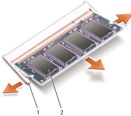
1 مشابك التثبيت (2) وحدة الذاكرة 2
