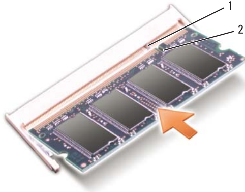
1 لسان 2 الشق
