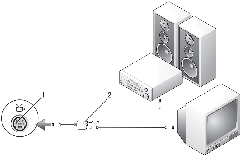
1 فتحة توصيل S-video TV-out 2 محول فيديو مركب
